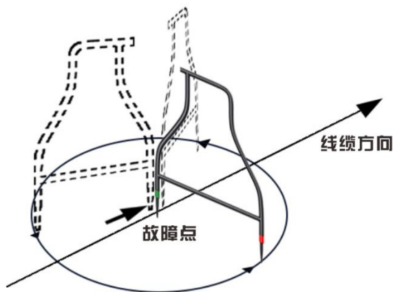
图 8-7 验证定位
