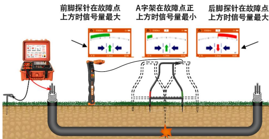
图 8-5 查障定点
