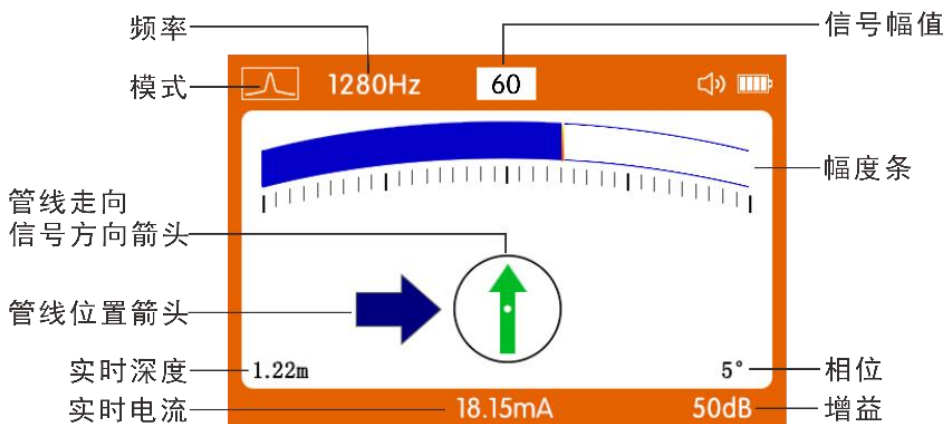
图 6-4 经典定位界面 (1)
