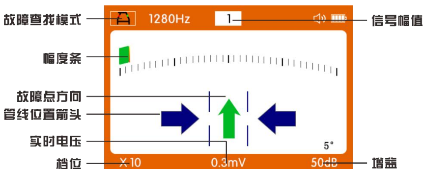
图 8-1 接收机故障查找界面
