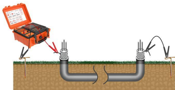
图 5-6 护层-大地接法接线图
