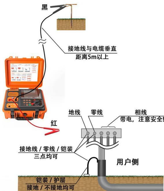
图 5- 20 运行电缆零线 / 地线 / 护层注入法
