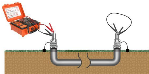
图 5-11 相间接法接线图
