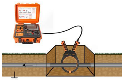
图 5-14 卡钳耦合接线图
